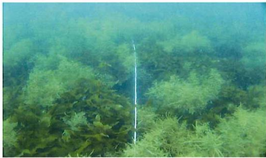
調査測線 6 水深10m周辺 被度 クロメ他 1 種：40~60%程度、ノギリモク他 5 種：30~60%程度
