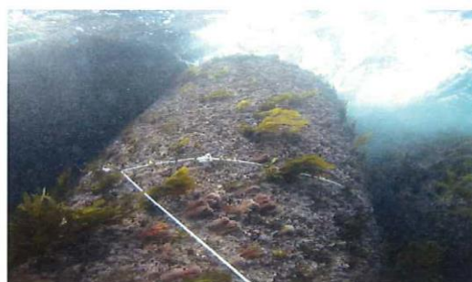
調査測線 4 水深 0 m 周辺 被度 加メ他 1 種 : 40% 程度
