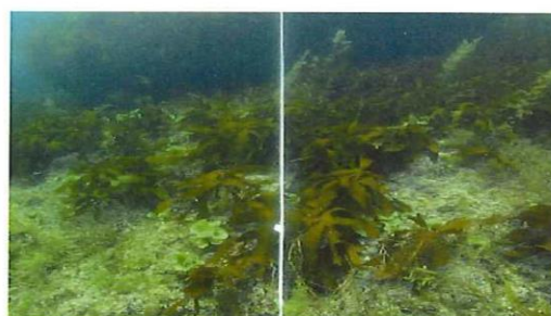
調査測線10 水深 4 m 周辺 被度 カメ他 1 種 : 60% 程度、ノギリ他 5 種 : 5% 未満
