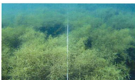
調査測線 4 水深 8 m 周辺 被度 加メ他 1 種 : 20~65% 程度、ノギリ他 5 種 : 30~90% 程度
